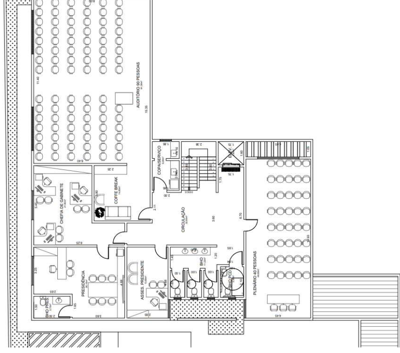
PLANTA BAIXA 2º PAVIMENTO - 294,82M 2
